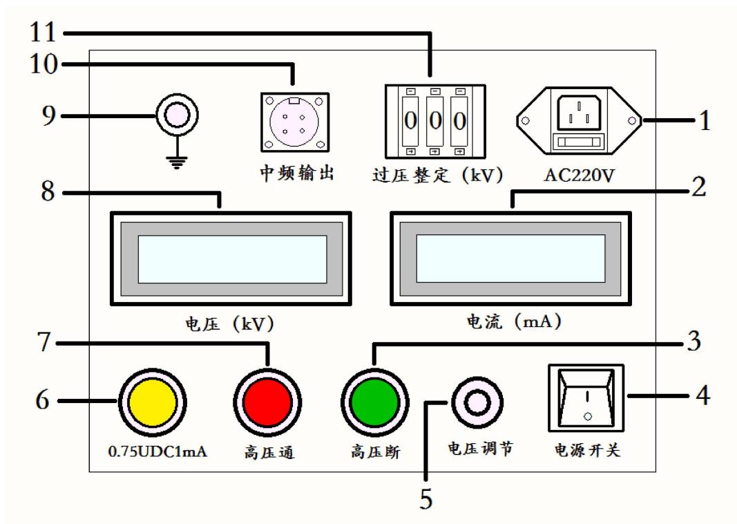
图 1.1 主机面板结构图
